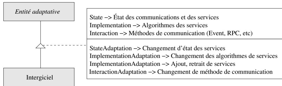
FIG. 5.24 – Modèle intergiciel par spécialisation d'entité adaptative
