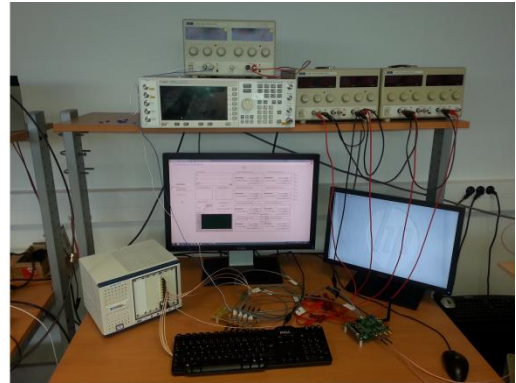
Figure 1 Synoptique de la plateforme de mesure de la consommation (gauche) et image de la plateforme utilisée pour la mesure de la consommation du front end Max2830
